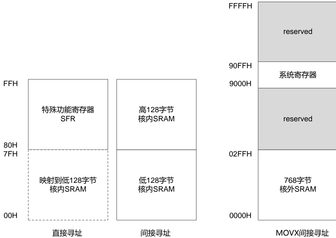
图表 12 数据寻址空间映射图
