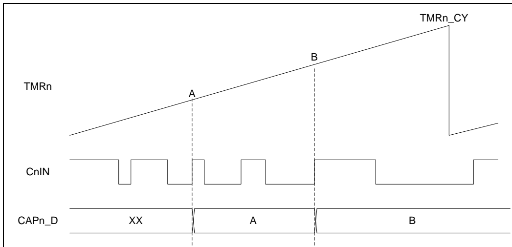
图表 20 捕捉累加模式示例波形图
