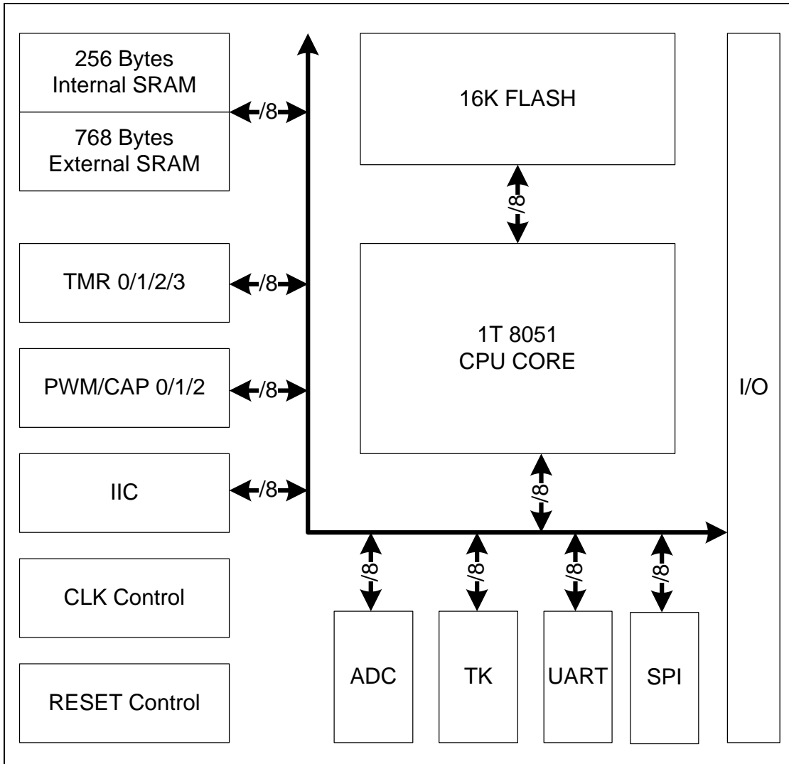
图表 7 E85F3325 功能框图
