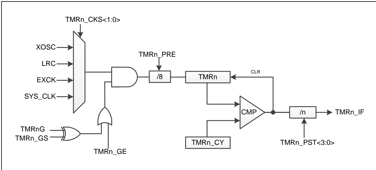
图表 17 TMR 功能框图
