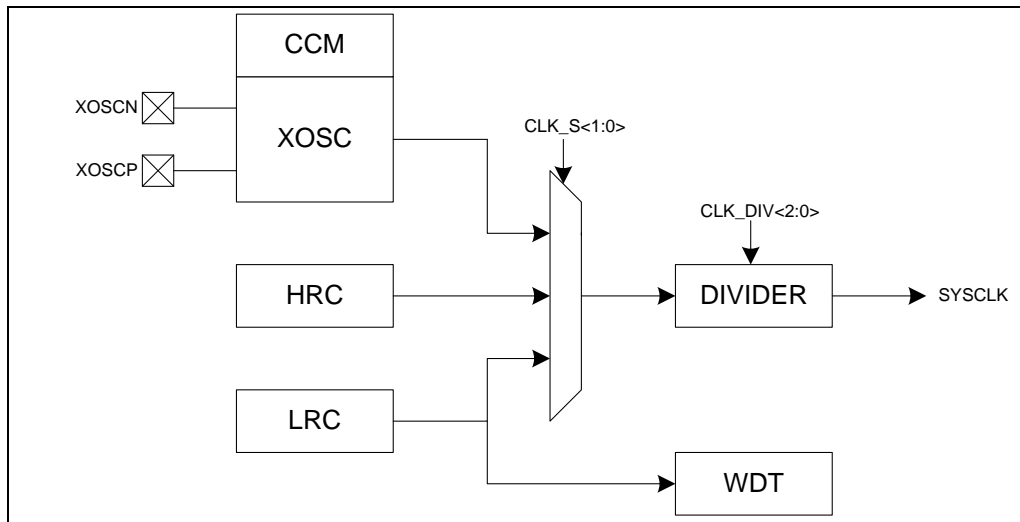
图表 13 系统时钟源功能框图
