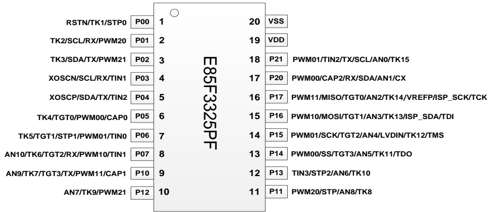
图表 1 SOP20 脚封装顶视图
