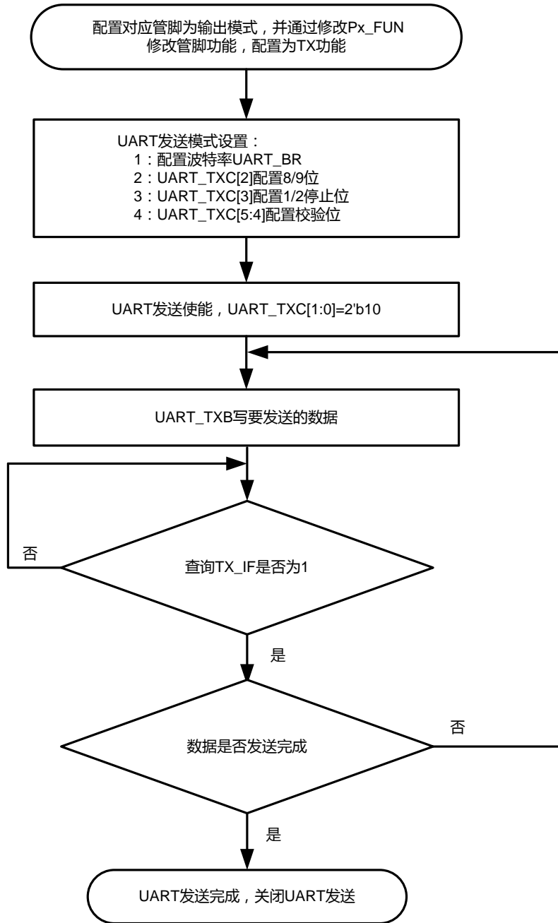
图表 25 UART 发送操作流程图
