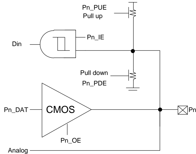
图表 16 I/O 功能框图
