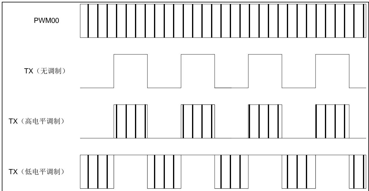
图表 24 UART 发送调制示意图
