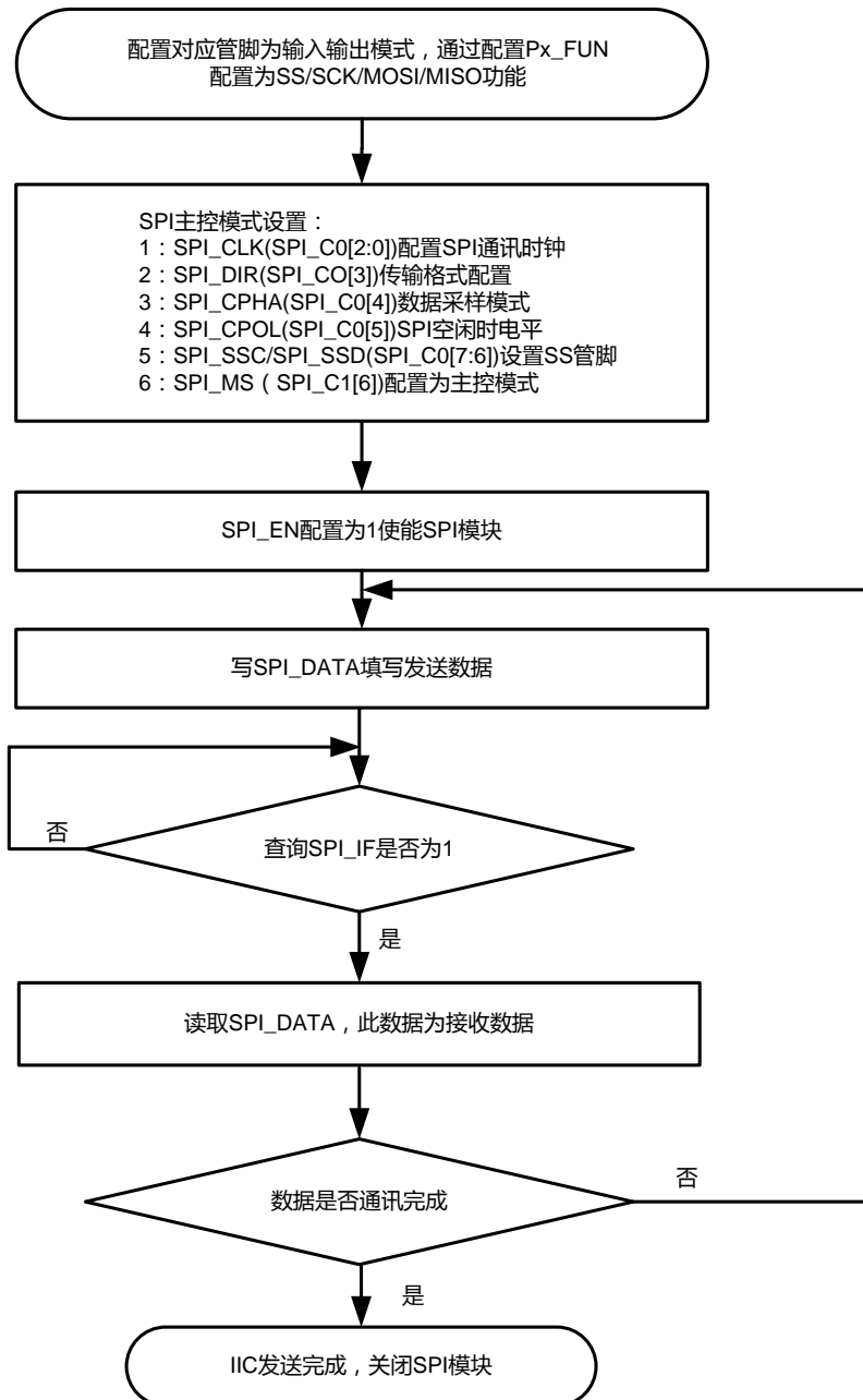
图表 30 SPI 主控模式流程图
