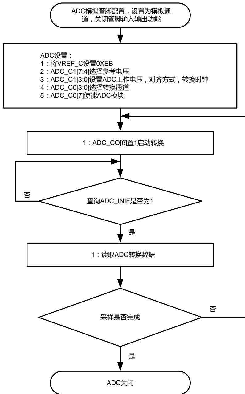
图表 32 ADC 操作流程
