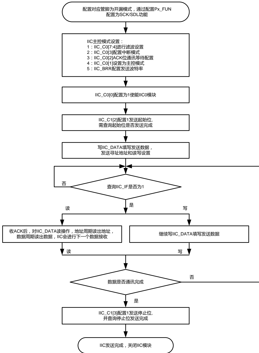
图表 28 IIC 主控通讯流程图
