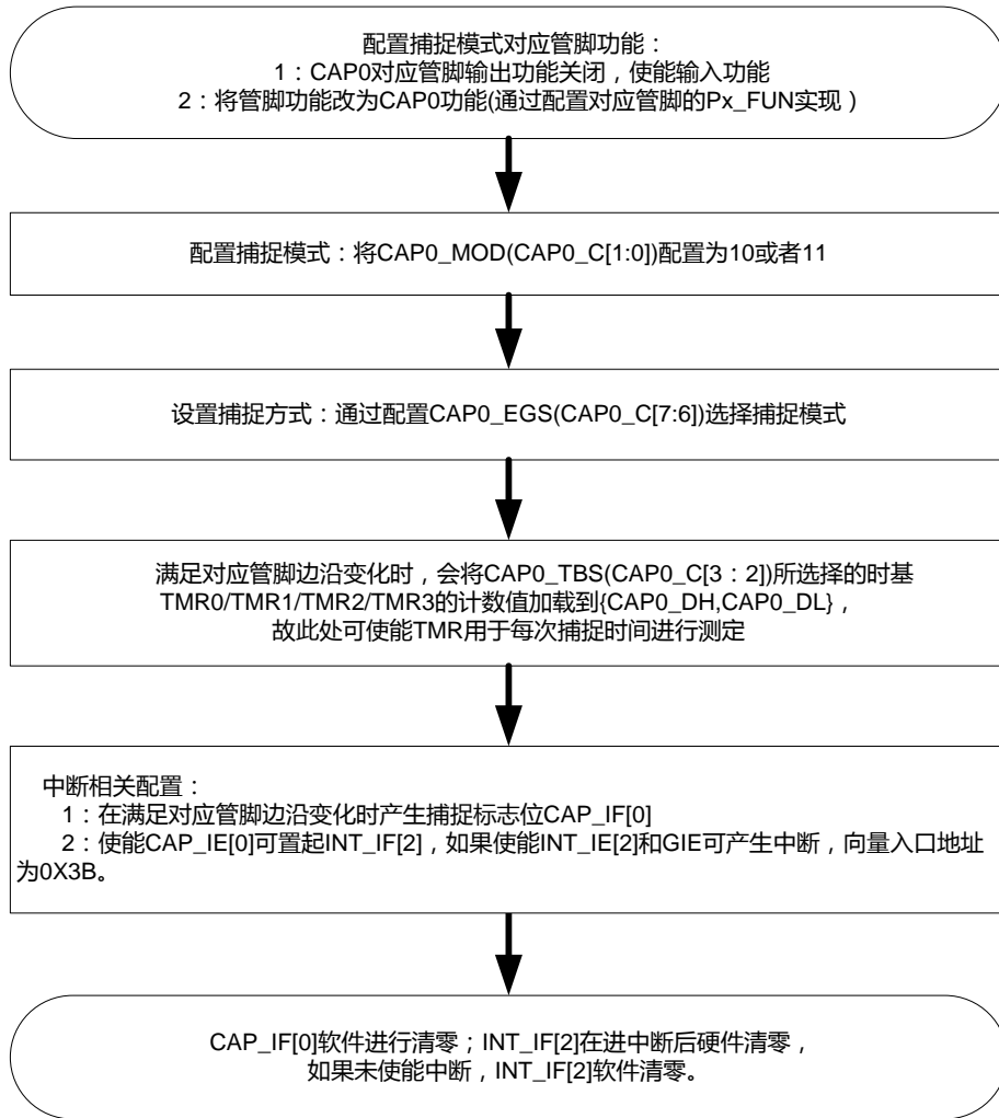
图表 21 CAP 操作流程图
