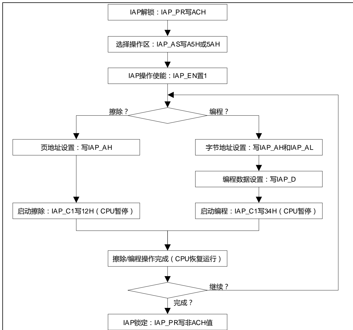
图表 11 IAP 操作流程图
