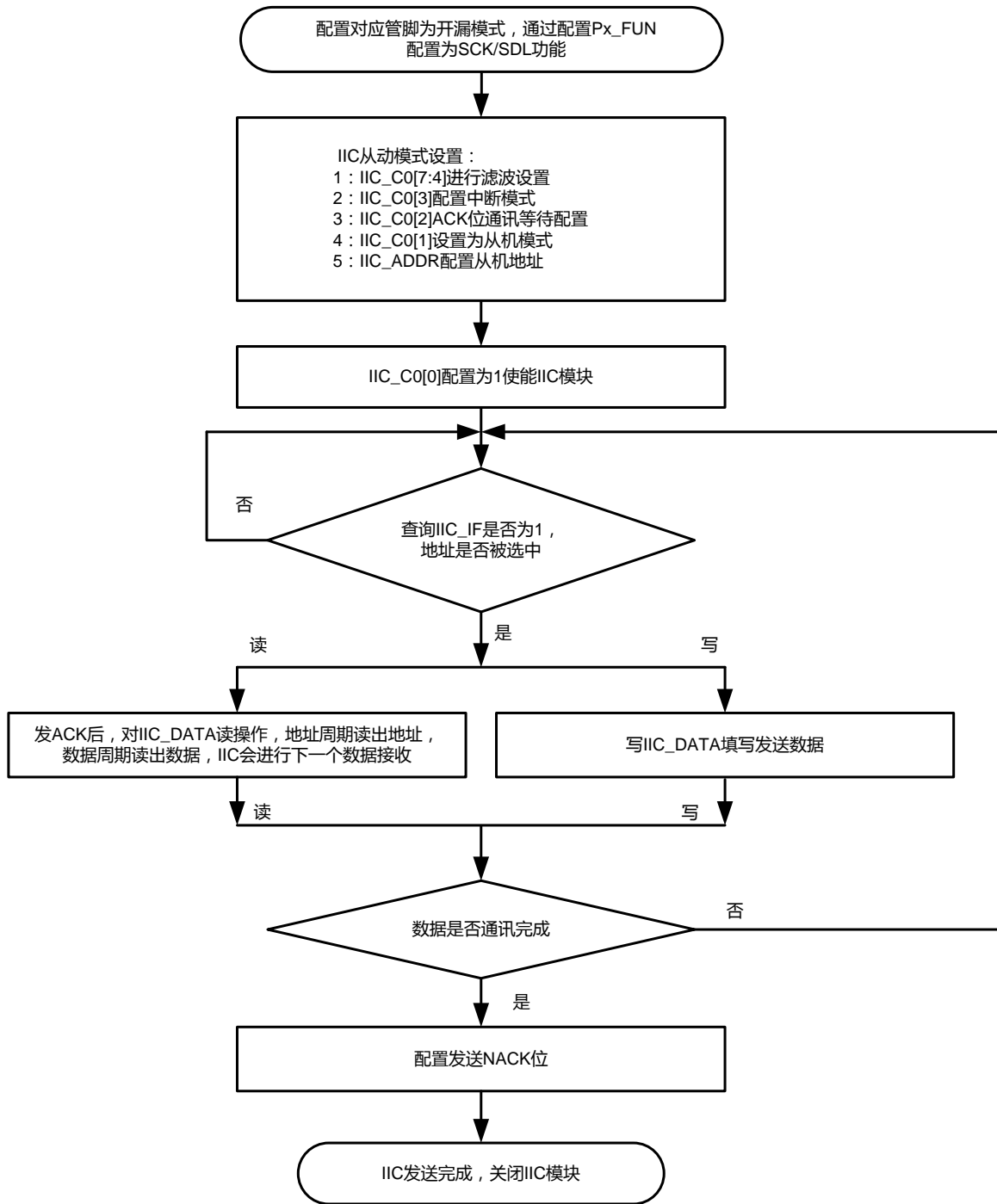
图表 29 IIC 从机通讯流程图
