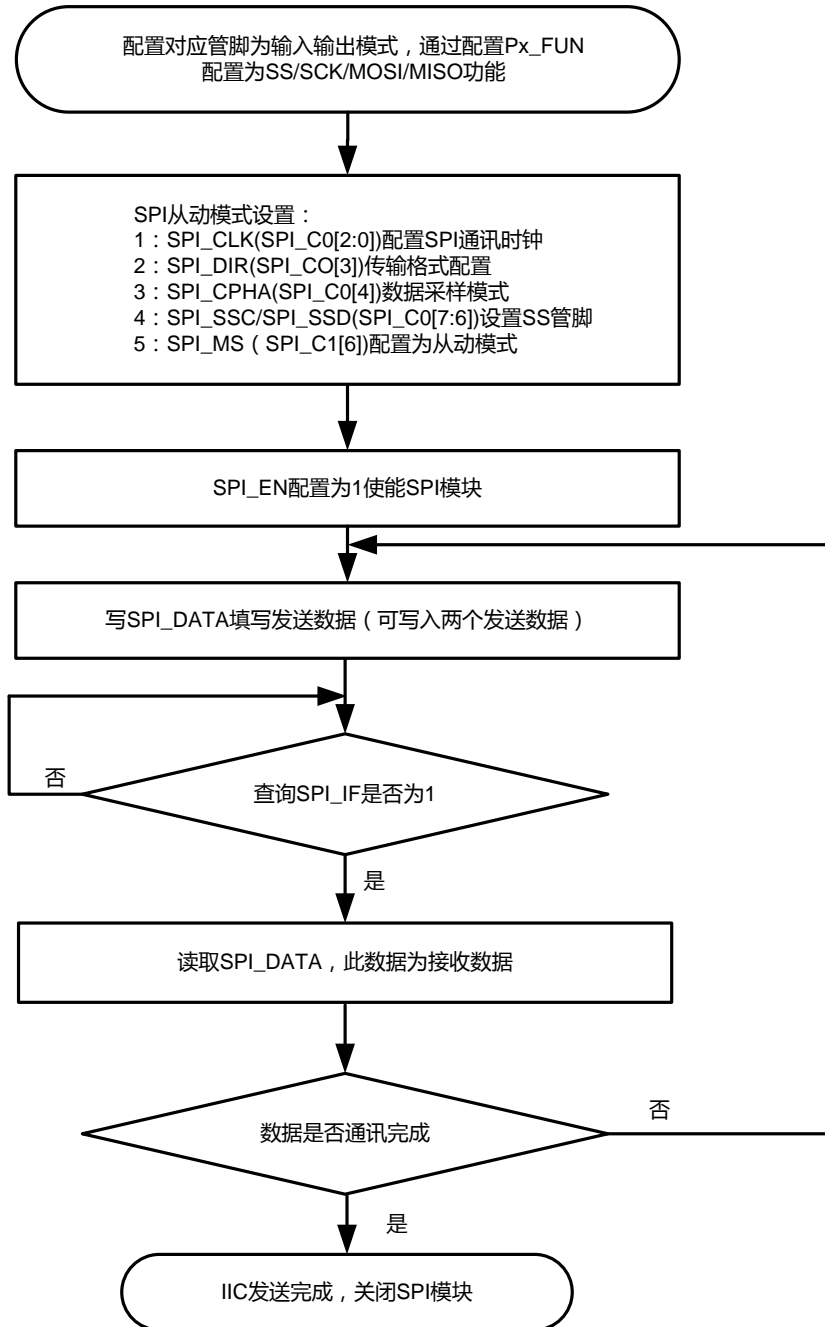
图表 31 SPI 从动模式流程图
