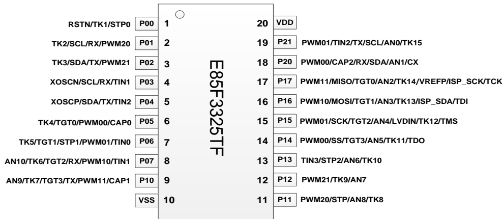
图表 2 TSSOP20 脚封装顶视图
