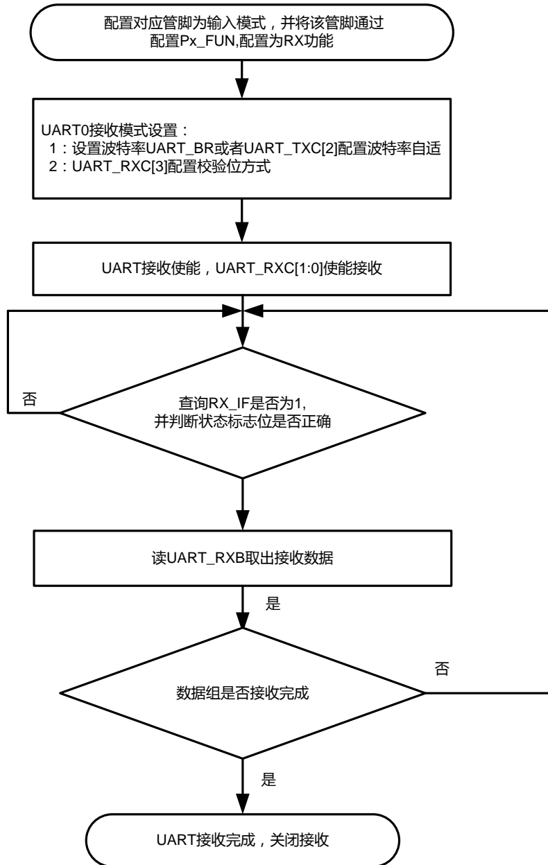
图表 26 UART 接收操作流程图
