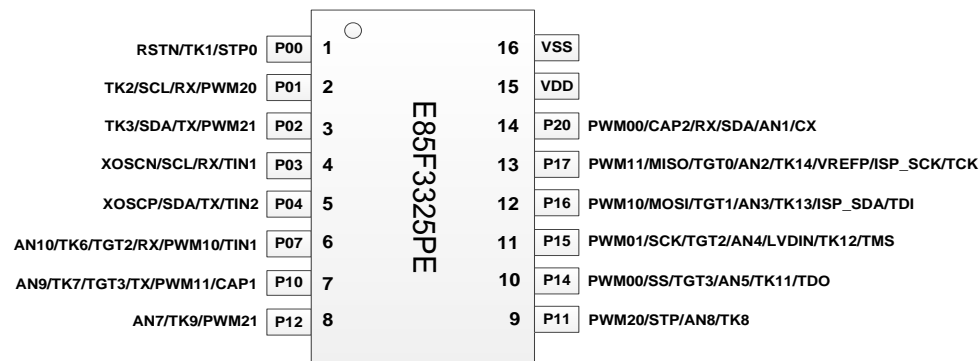
图表 3 SOP16 脚封装顶视图
