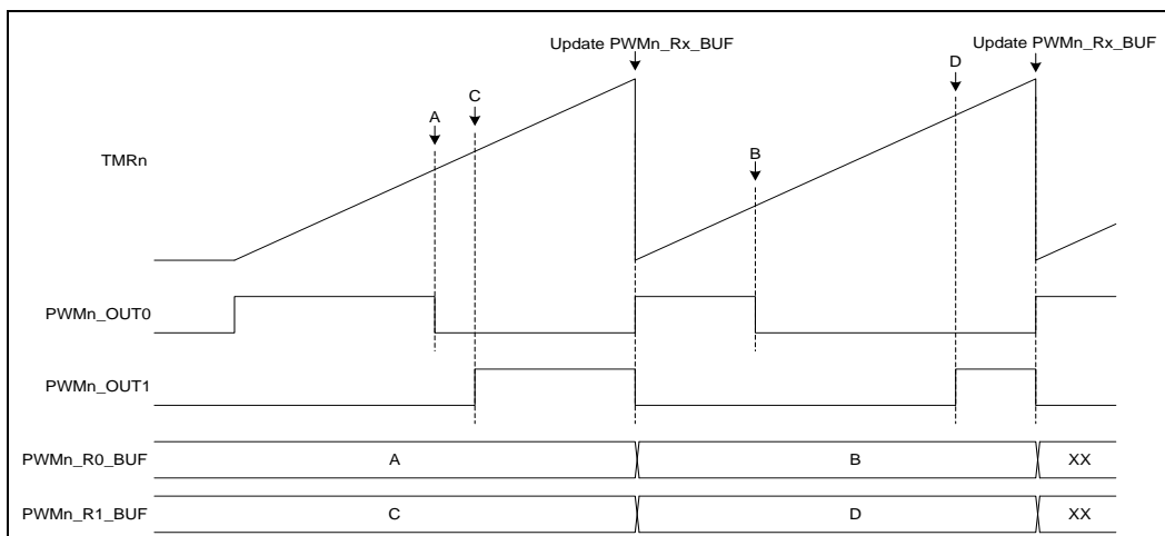
图表 22 PWM 工作示例波形图
