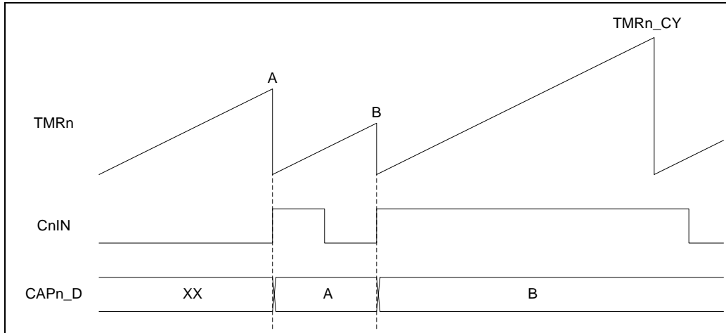
图表 19 捕捉清零模式示例波形图
