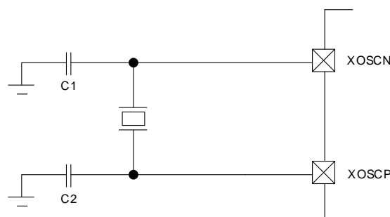
图表 14 外部振荡器 XOSC 连接示意图
