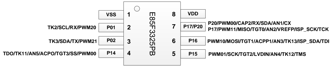
图表 4 SOP8 脚封装顶视图
