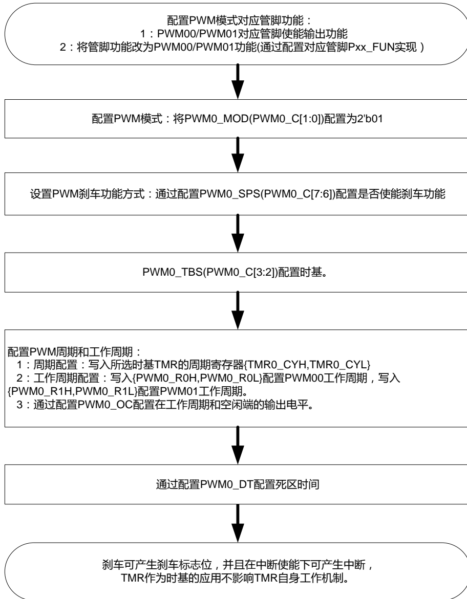
图表 23 PWM 操作流程图
