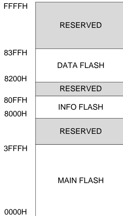
图表 8 程序存储空间映射图
