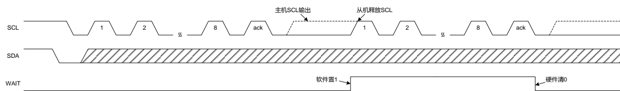
图表 27 IIC 通信等待波形示意图
