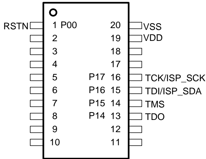
图表 10 ISP 复用端口定义图
