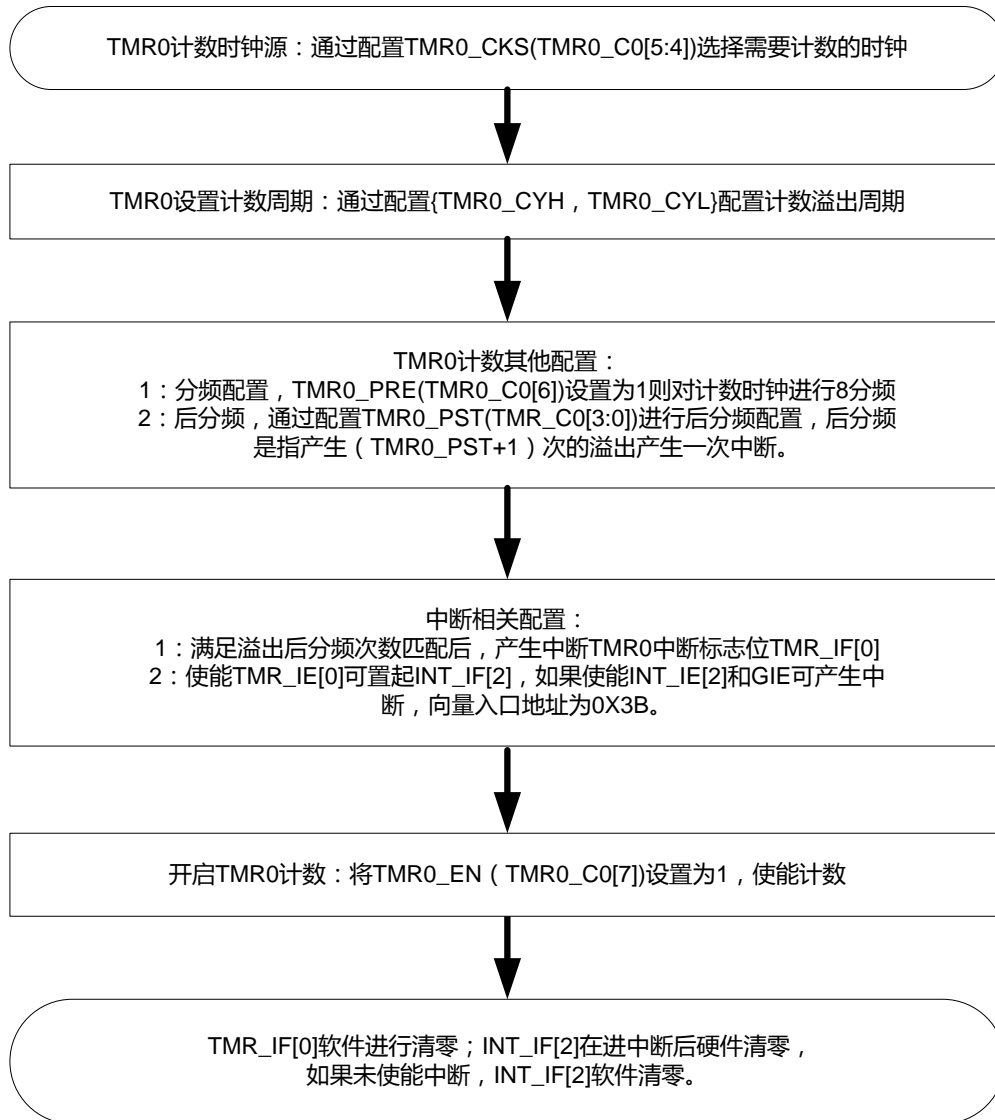
图表 18 TMR 操作流程图
